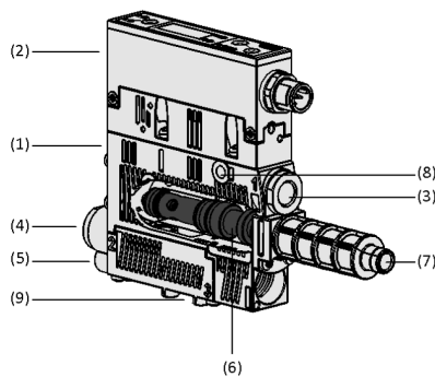
Systemaufbau Kompaktejektoren SCPS- / SCPSb- / SCPSi-UHV-HD
