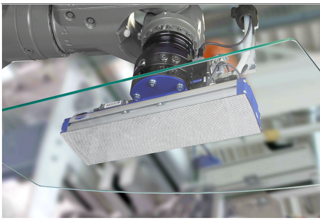
Sistema di presa FXP con strato protettivo SU per la movimentazione del vetro
