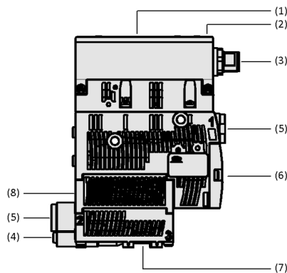
Systemaufbau Kompaktejektoren SCPSc / SCPSi
