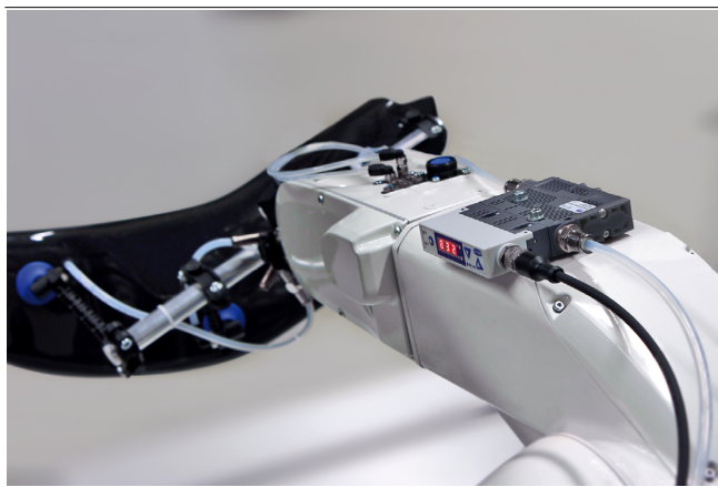
Zentrale Vakuum-Erzeugung durch Kompaktejektoren SCPSi
