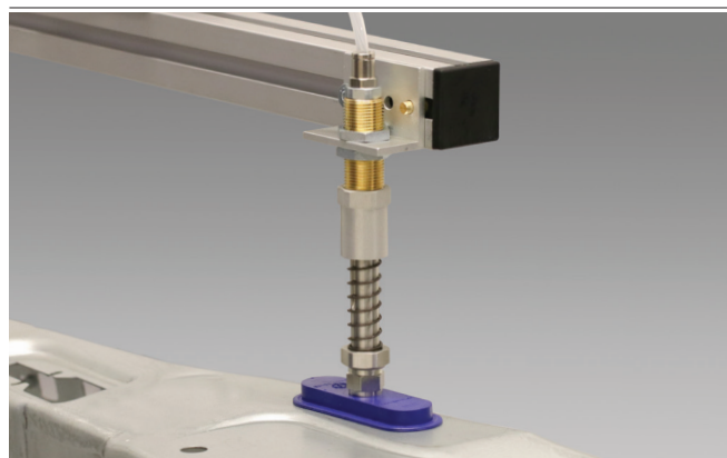
Aste a molla FSTE-HDB per la movimentazione di lamiere grezze da costruzione
