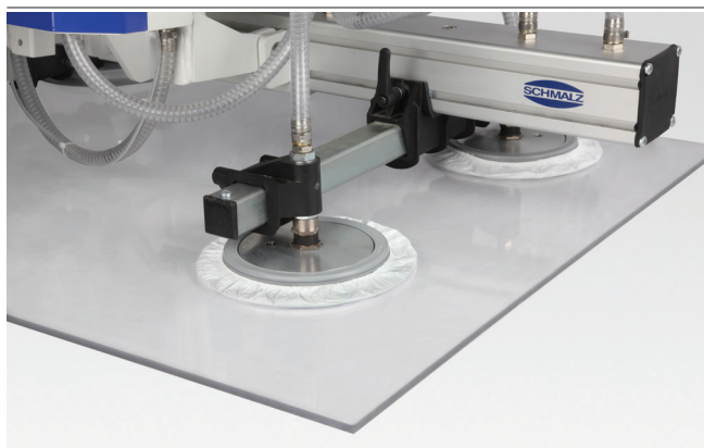
Rivestimenti ventose SU per la movimentazione di lastri di vetro delicati
